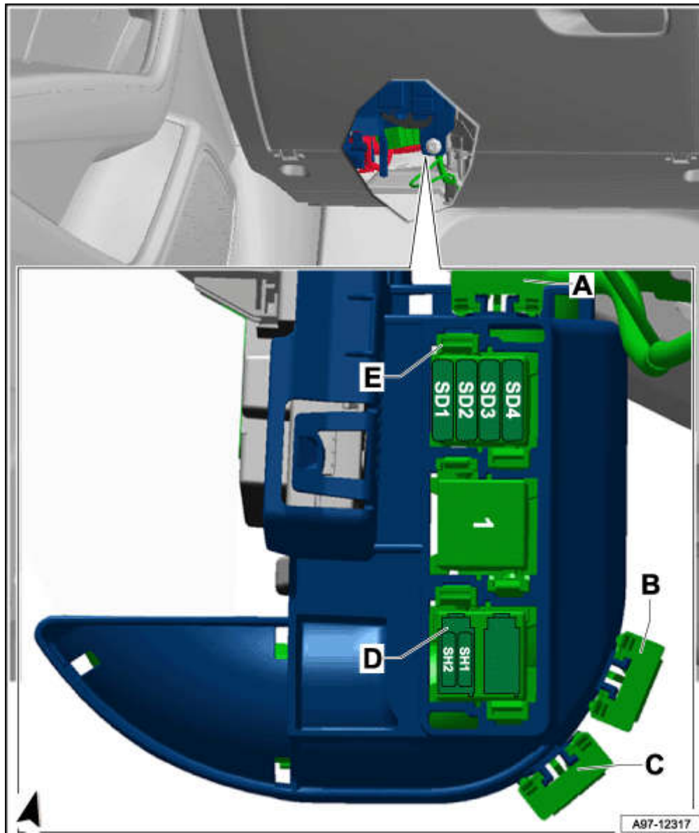
1 - 继电器 -J989-
